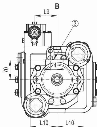
PVH90, PVH112
