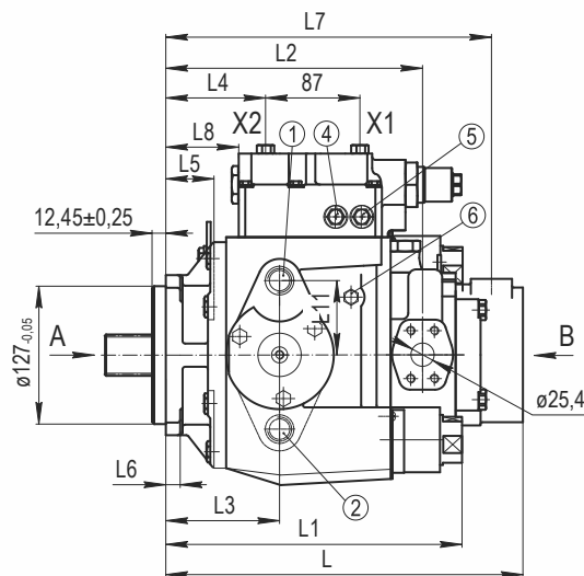
PVH71
