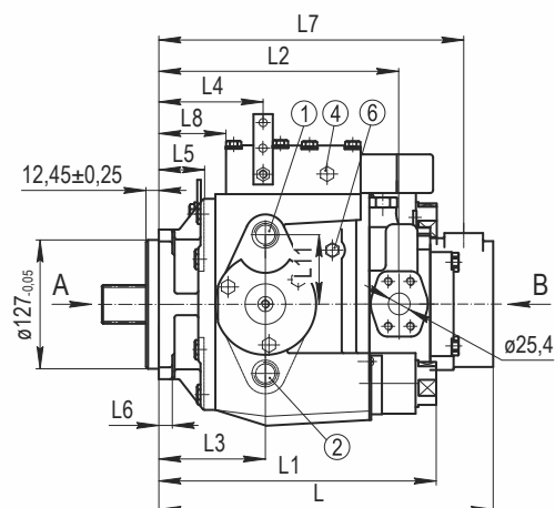
PVH71
