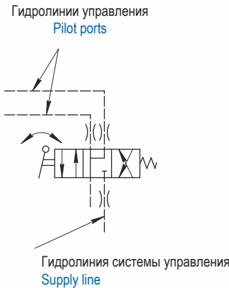
Схема распределителя с жиклерами Control valve with orifice
