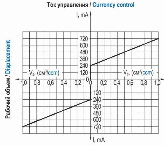
График зависимости на 24V 24V dependency graph
