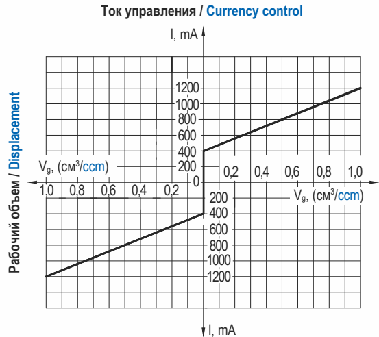
График зависимости на 12V 12V dependency graph
