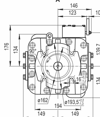
PVH90, PVH112
