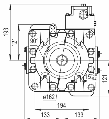
PVH71
