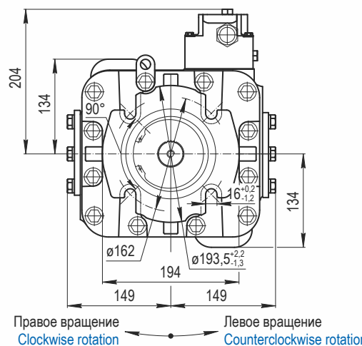
PVH90, PVH112
