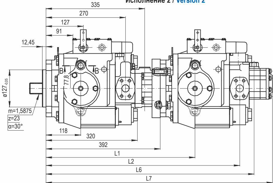
Исполнение 2 / Version 2
