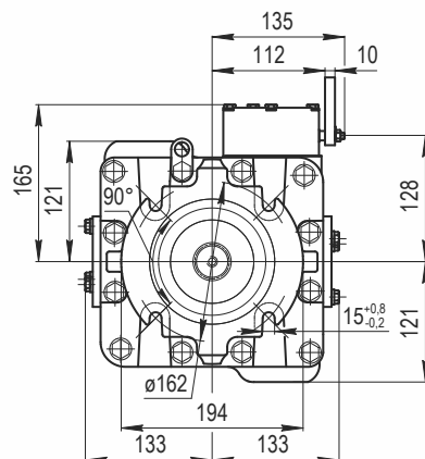
PVH71
