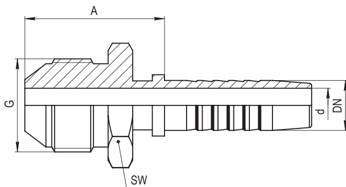
Штуцер типа CJIC37° (конус 74°) CJIC 37° MALE 74° cone
