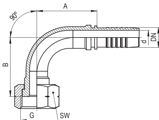
Ниппель типа ORFS 90° 90° ORFS FEMALE
