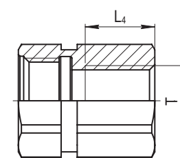
Резьбовое соединение Threaded connection
