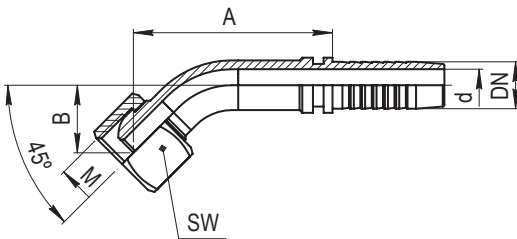
Ниппель типа DKM 45° (сфера под штуцер с углом 60°) DKM FEMALE 60° SPHERE
