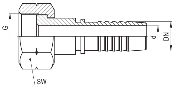
Ниппель типа ORFS ORFS FEMALE
