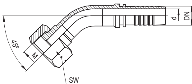
Ниппель типа ORFS 45° 45° ORFS FEMALE
