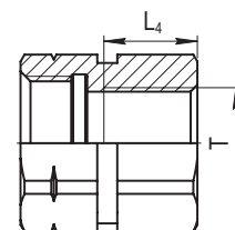
Резьбовое соединение Threaded connection
