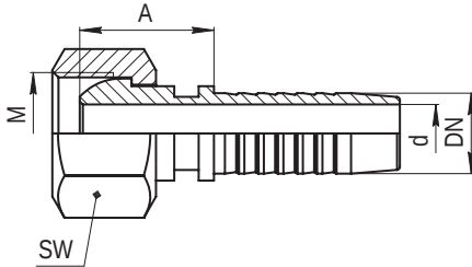
Ниппель типа DKM (сфера под штуцер с углом 60°) DKM FEMALE 60° SPHERE
