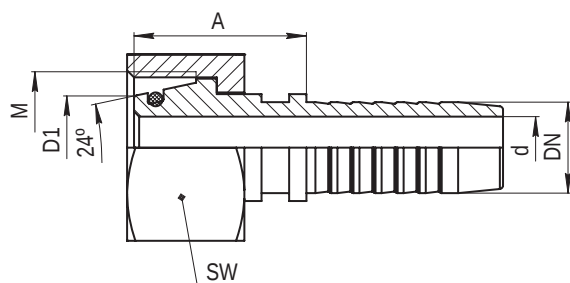
Ниппель типа DKOL легкая серия (конус 24° с резиновым уплотнением) DKOL Femaly 24° cone o-ring
