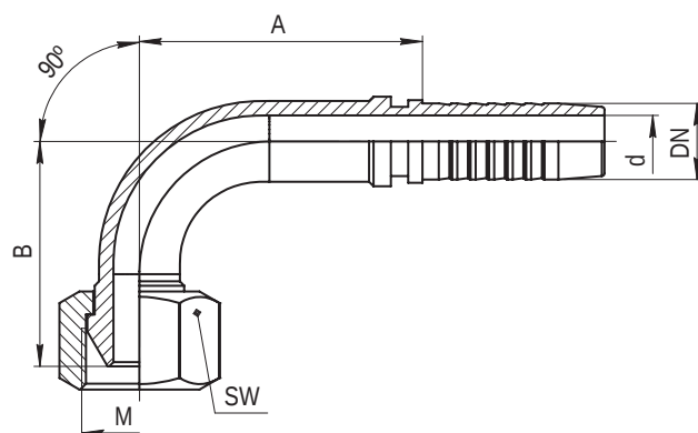
Ниппель типа DKR 90° (конус 60°) 90° DKR FEMALE 60° CONE
