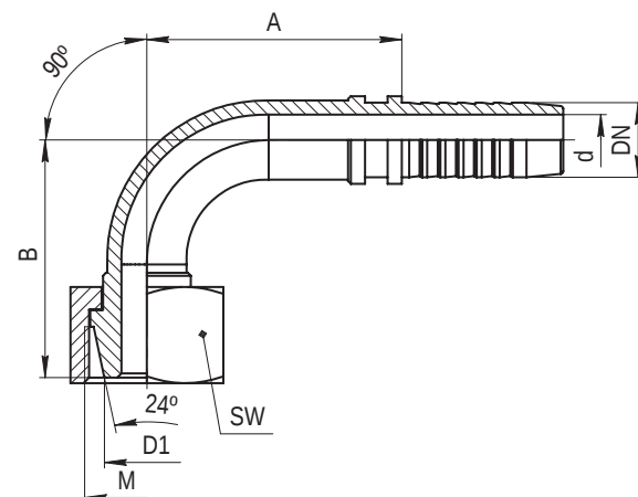
Ниппель типа DKS 90° тяжелая (S) серия (конус 24°) 90° DKS Femaly 24° cone
