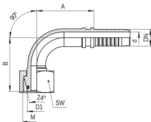
Ниппель типа 90° DKOL легкая серия (конус 24° с резиновым уплотнением) 90° DKOL Femaly 24° cone o-ring
