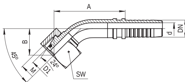
Ниппель типа 45° DKOL легкая серия (конус 24° с резиновым уплотнением) 45° DKOL Femaly 24° cone o-ring
