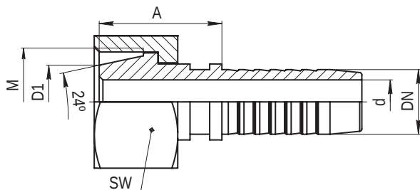
Ниппель типа DKS тяжелая (S) серия (конус 24°) DKS Femaly 24° cone
