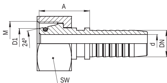
Ниппель типа DKOS легкая серия (конус 24° с резиновым уплотнением) DKOS Femaly 24° cone o-ring
