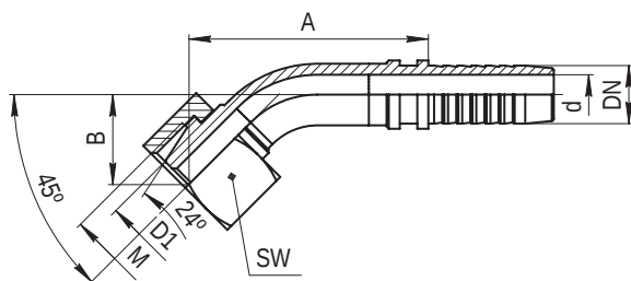
Ниппель типа DKS 45° тяжелая (S) серия (конус 24°) 45° DKS Femaly 24° cone
