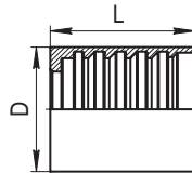
Муфта типа Е (для продольной обжимки) Ferrule E type
