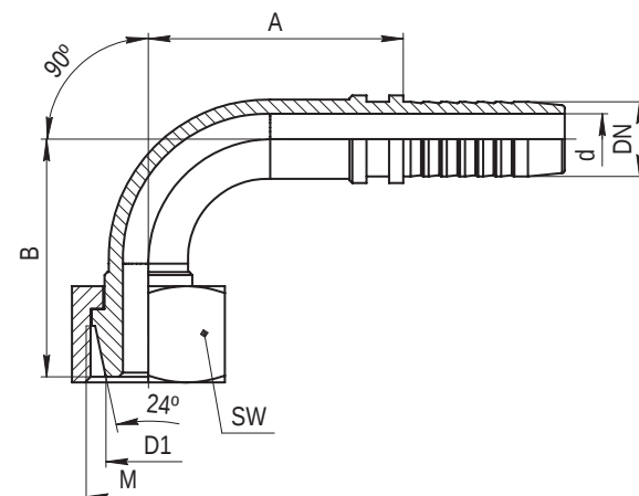
Ниппель типа DKL 90° легкая (L) серия (конус 24°) 90° DKL Femaly 24° cone
