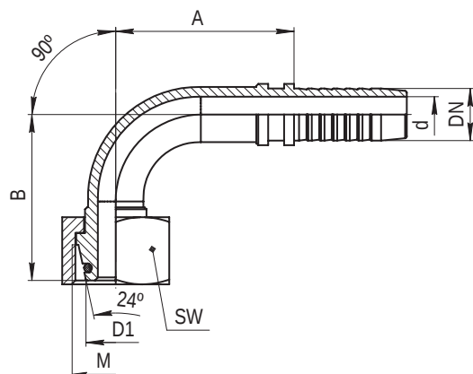
Ниппель типа 90° DKOS тяжелая серия (конус 24° с резиновым уплотнением) 90° DKOS Femaly 24° cone o-ring
