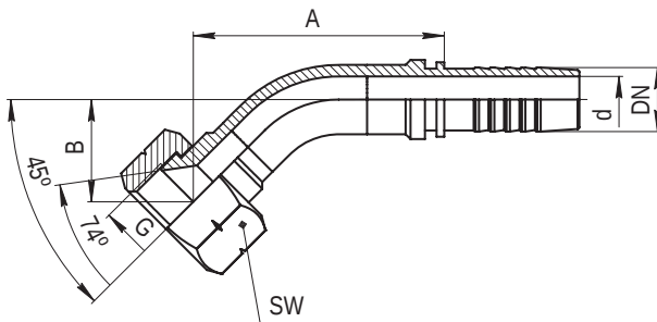
Ниппель типа JIC 37°-45 (конус 74°) JIC 37°-45 Female 74° cone
