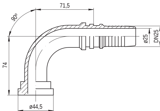
Ниппель SFL3-1"-90°-DN25 90° SFL3-1" Famele DN 25
