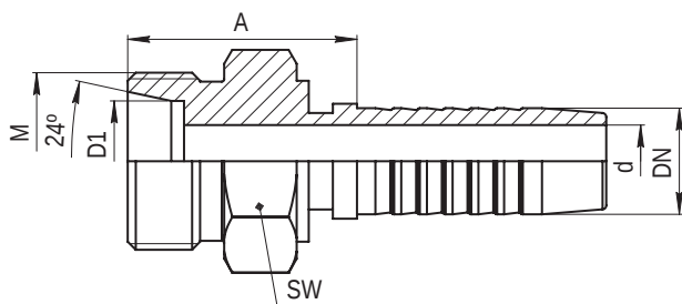
Штуцер типа CES тяжелая серия (конус 24°) CES Femaly 24° cone
