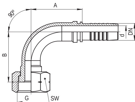
Ниппель типа ORFS 90° 90° ORFS Femaly
