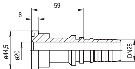
Ниппель SFL3-1"-DN 25 SFL3-1" Famele DN 25
