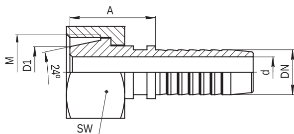
Ниппель типа DKL легкая (L) серия (конус 24°) DKL Femaly 24° cone
