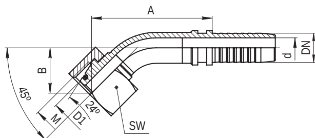
Ниппель типа 45° DKOS тяжелая серия (конус 24° с резиновым уплотнением) 45° DKOS Femaly 24° cone o-ring
