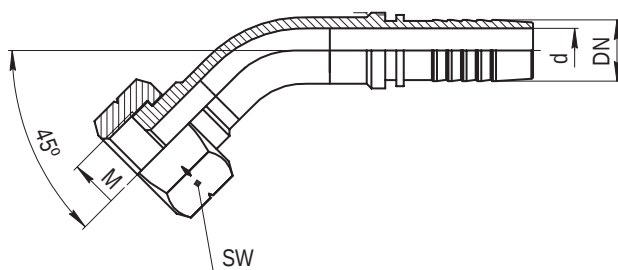
Ниппель типа ORFS 45° 45° ORFS Femaly
