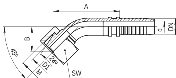
Ниппель типа DKL 45° легкая (L) серия (конус 24°) 45° DKL Femaly 24° cone
