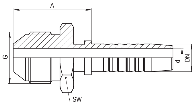
Штуцер типа CJIC37° (конус 74°) CJIC 37° Femaly 74° cone
