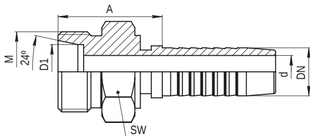
Штуцер типа CEL легкая серия (конус 24°) CEL Femaly 24° cone
