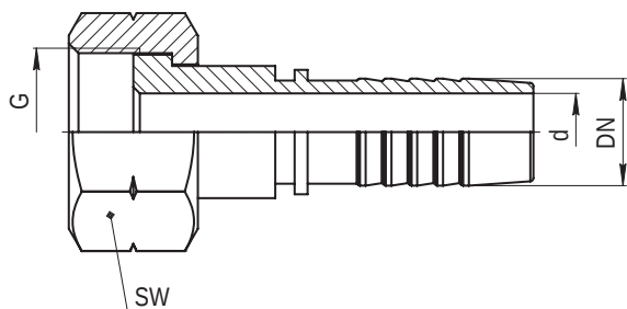
Ниппель типа ORFS ORFS Femaly
