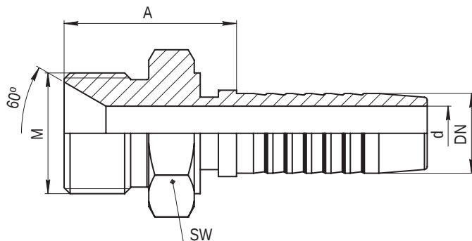
Штуцер типа СМ (конус 60°) CM Femaly 60° cone
