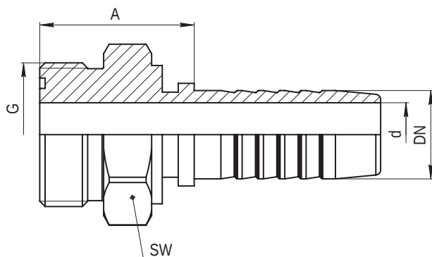
Штуцер типа CORFS CORFS Femaly
